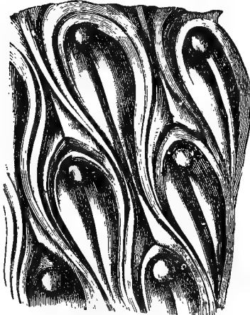
LEPIDODENDRON OBOVATUM. (Nat. size.)
